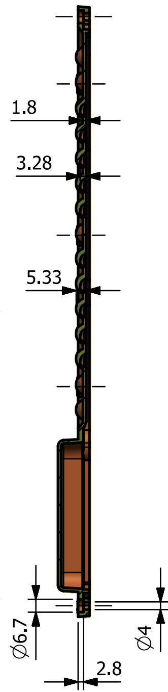
SECTION A-A
